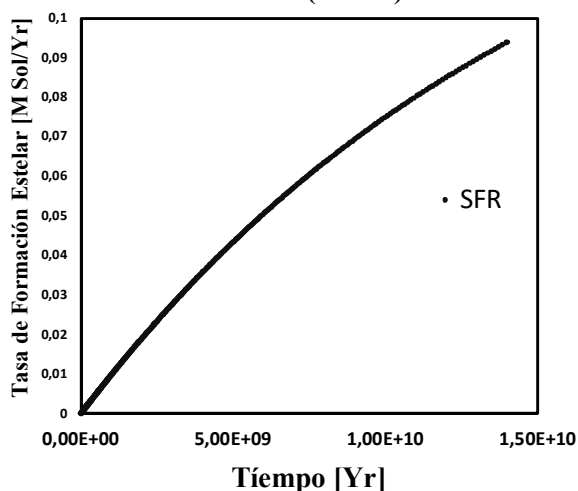
Figura 6. Gráfica de la tasa de formación estelar SFR (ordenada) contra el tiempo (abscisa).
